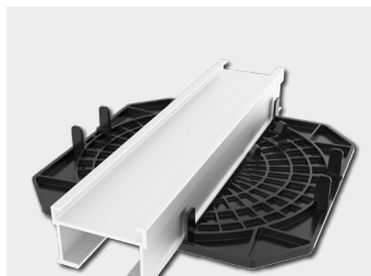
Lastverteilplatte + Alu-Profil
