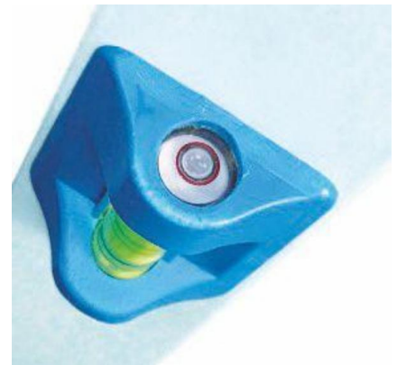
Mit zwei Libellen zur Kontrolle von horizontalen und vertikalen Messungen
